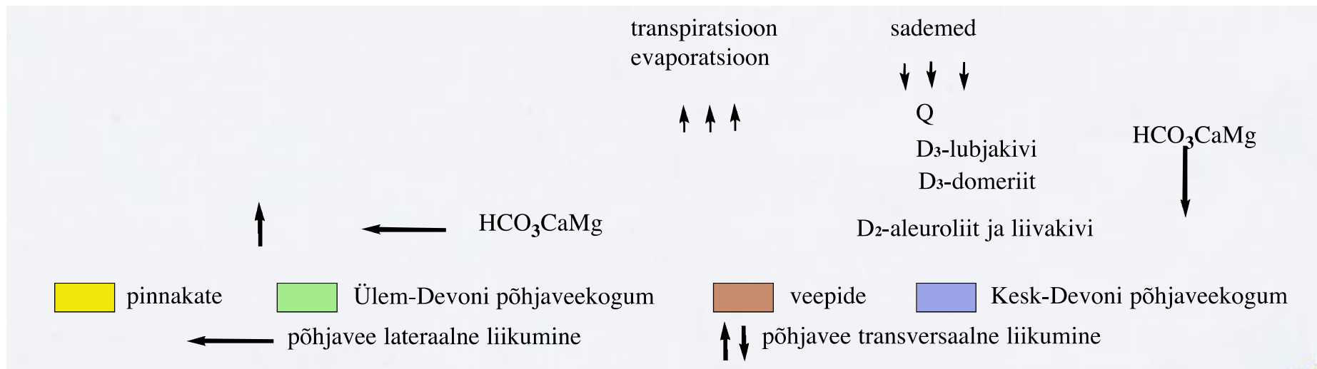
Joonis 3. Ülem-Devoni ja Kesk-Devoni põhjaveekogumite kontseptuaalse mudeli visualiseeritud läbilõige Koiva vesikonnas (Autor: OÜ Eesti Geoloogiakeskus, 2012).
