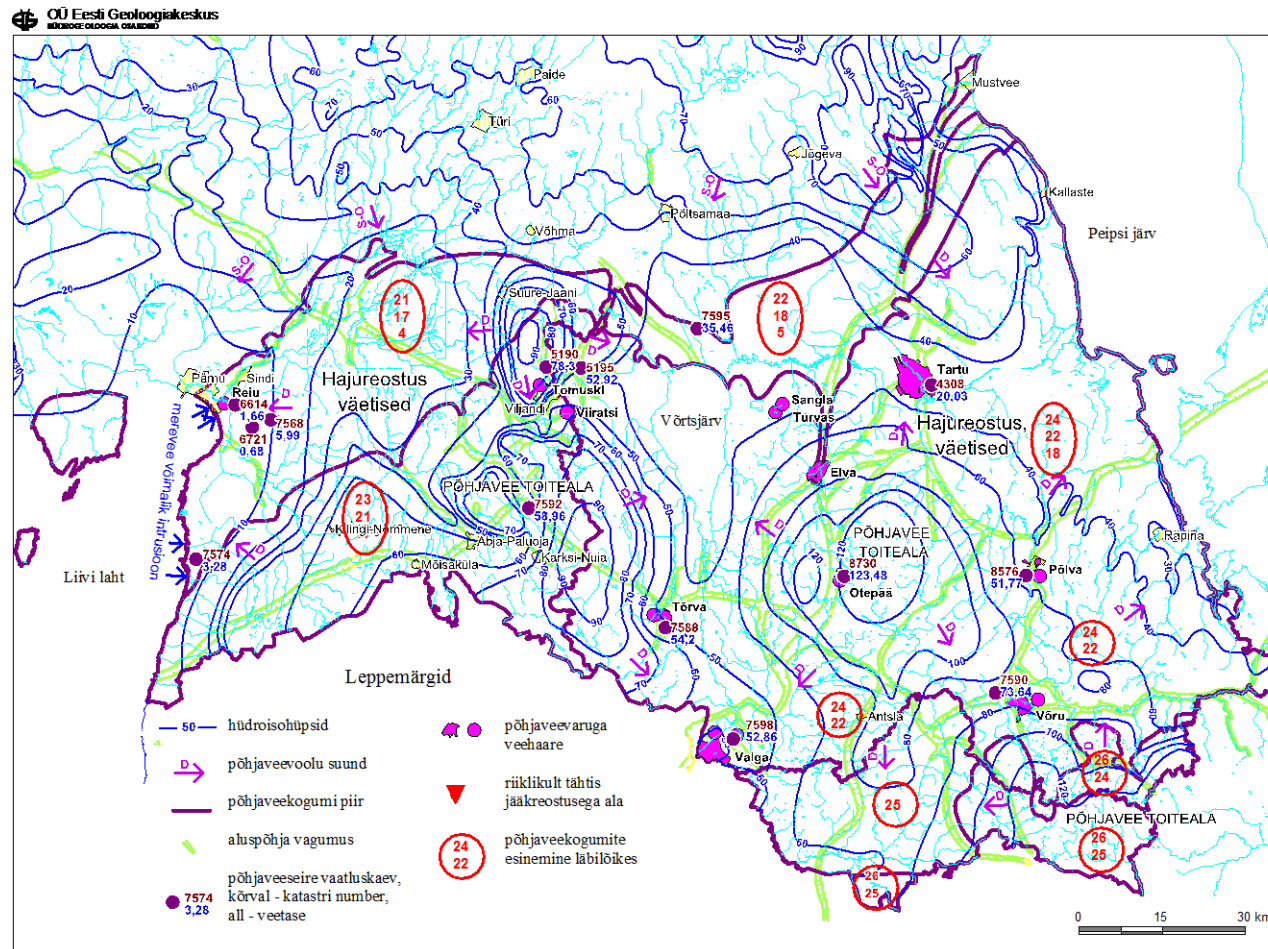
Joonis 1. Devoni põhjaveekogumite visualiseeritud kontseptuaalne mudel (Autor: OÜ Eesti Geoloogiakeskus, 2012).
